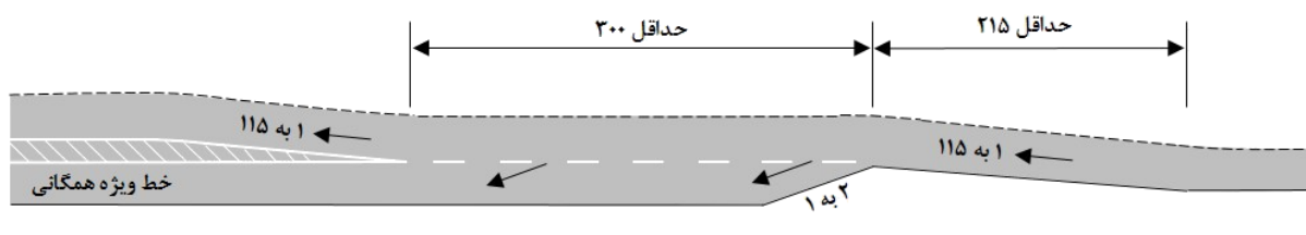
شکل ۷-۴- مشخصات هندسی ابتدای خط ویژه میانی جدا شده با خط‌کشی (کلیه مقادیر به متر است)
