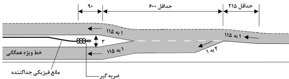
شکل ۷-۵- مشخصات هندسی ابتدای خط ویژه میانی جدا شده با موانع فیزیکی (کلیه مقادیر به متر است)
